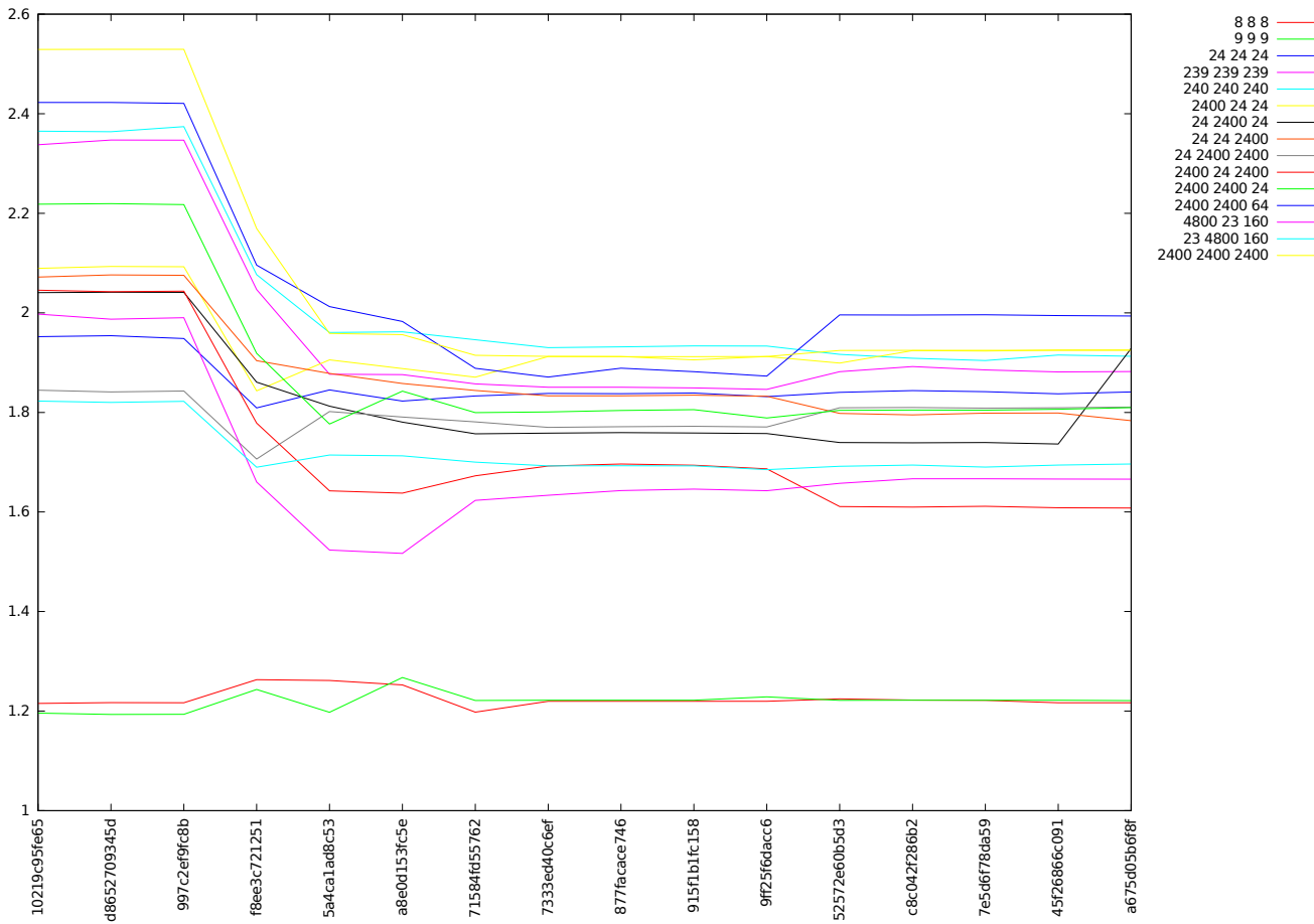
nehalem-sse4-cgemm
